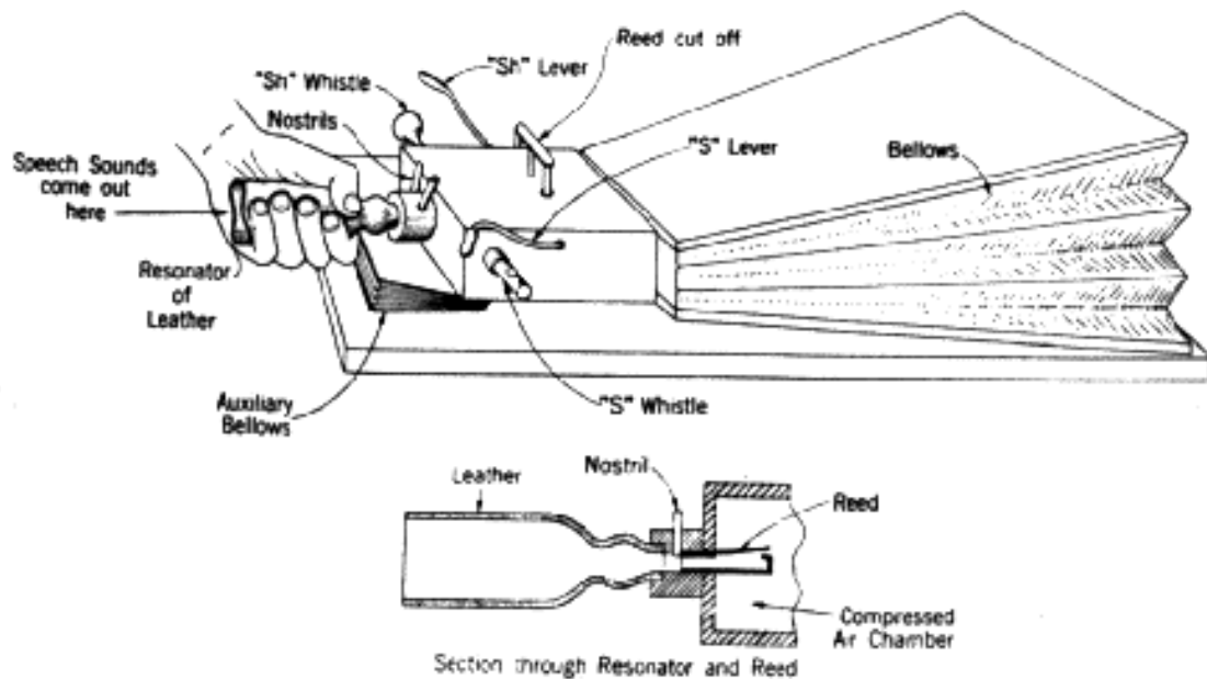
Fig. 3: Máquina parlante de Wheatstone (Reproducida de Dudley y Tarnockzy, 1950)
