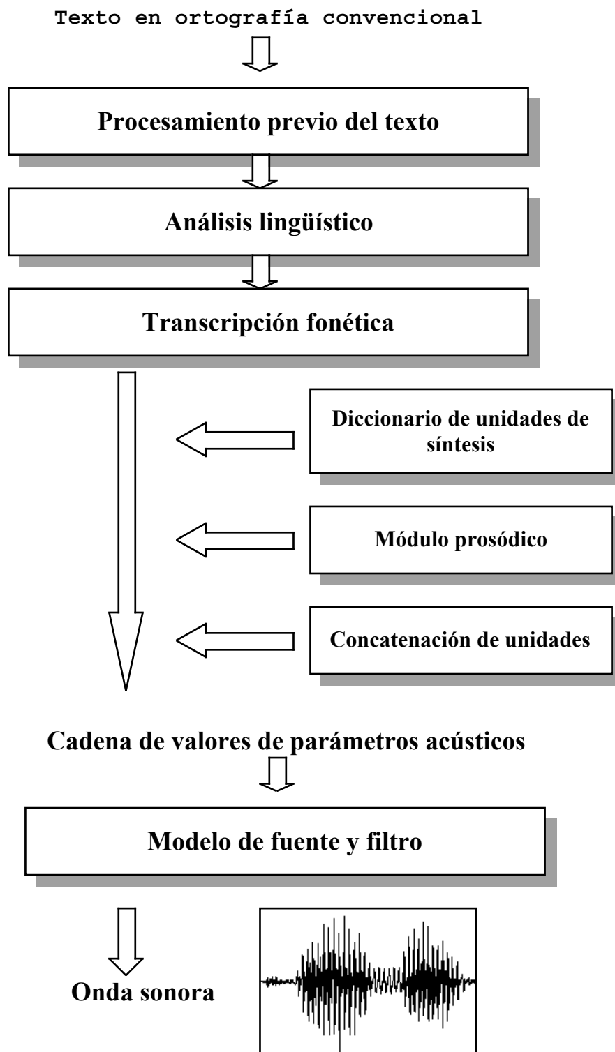
Figura 8: Esquema simplificado del proceso de conversión de texto en habla
